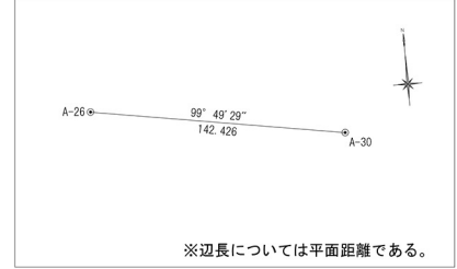
第VI系・平均縮尺係数 (0.999912)
